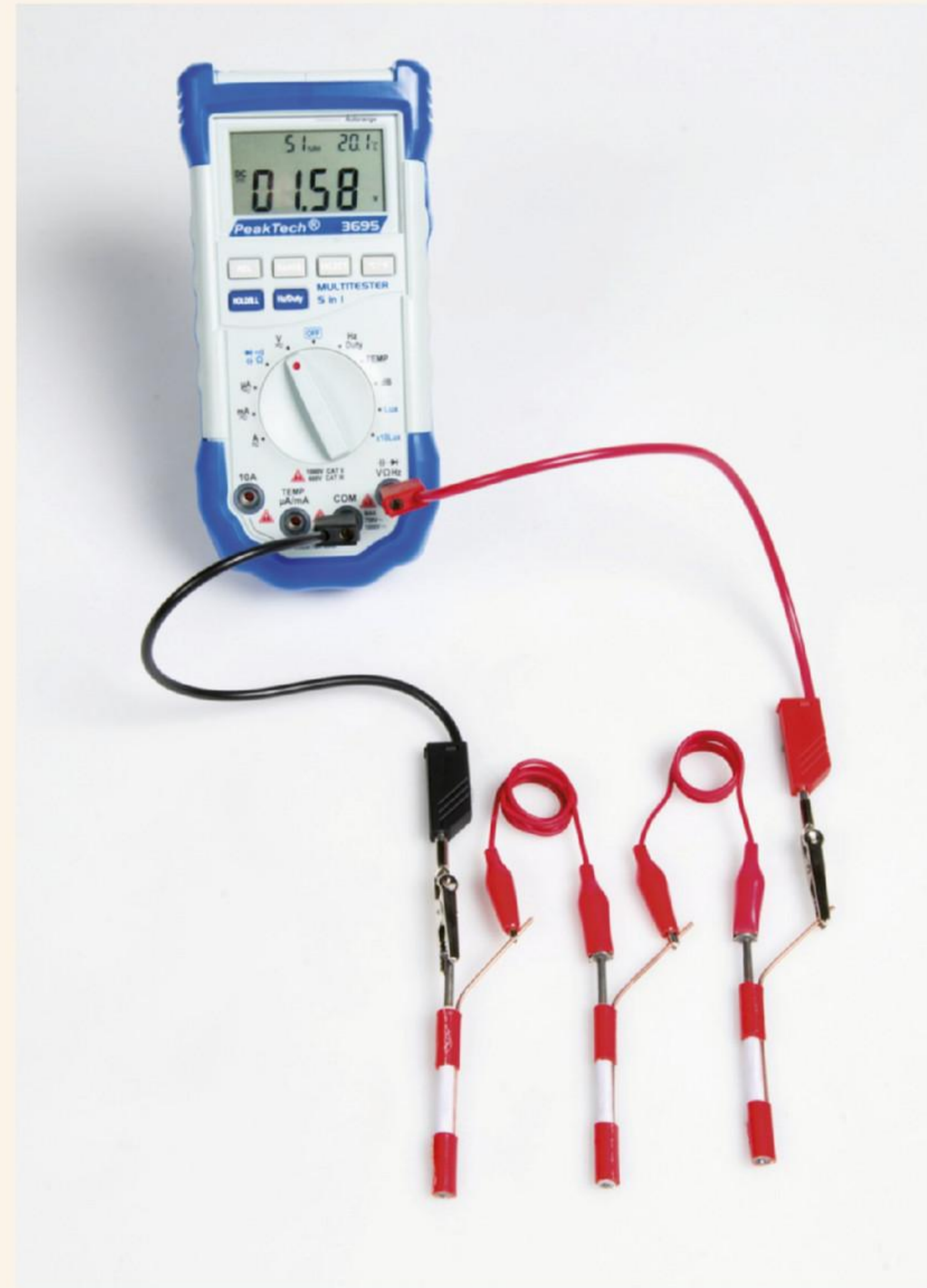
afbeelding 21 Drie batterijen aangesloten op de voltmeter.
