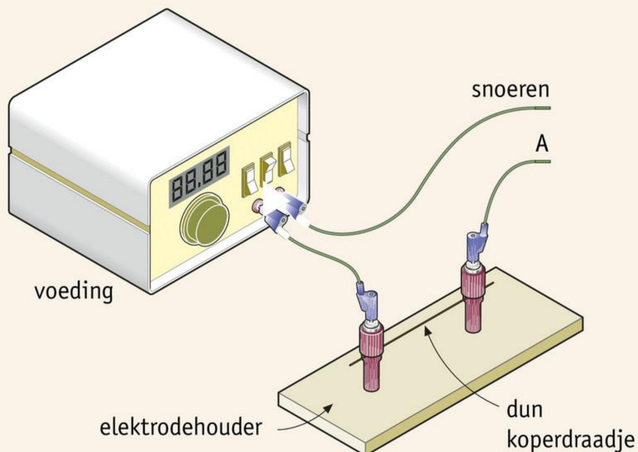
afbeelding 11 De aansluiting van proef 8.
