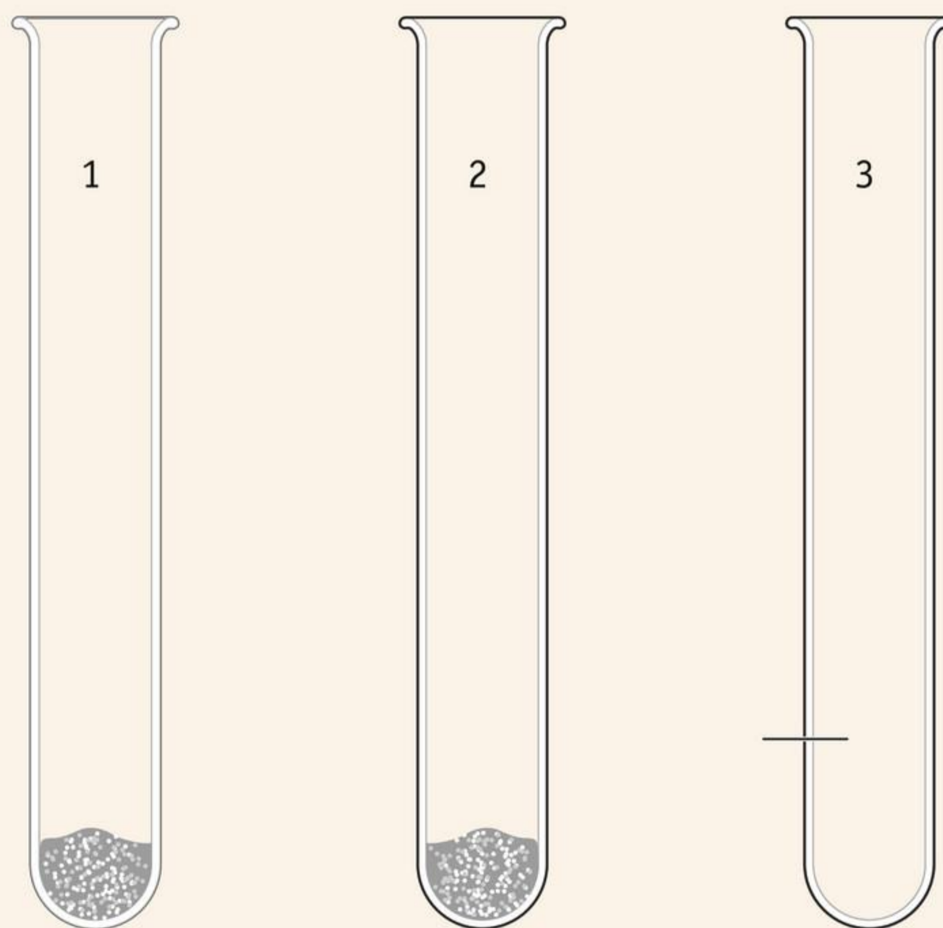
afbeelding 5 Drie reageerbuizen.
