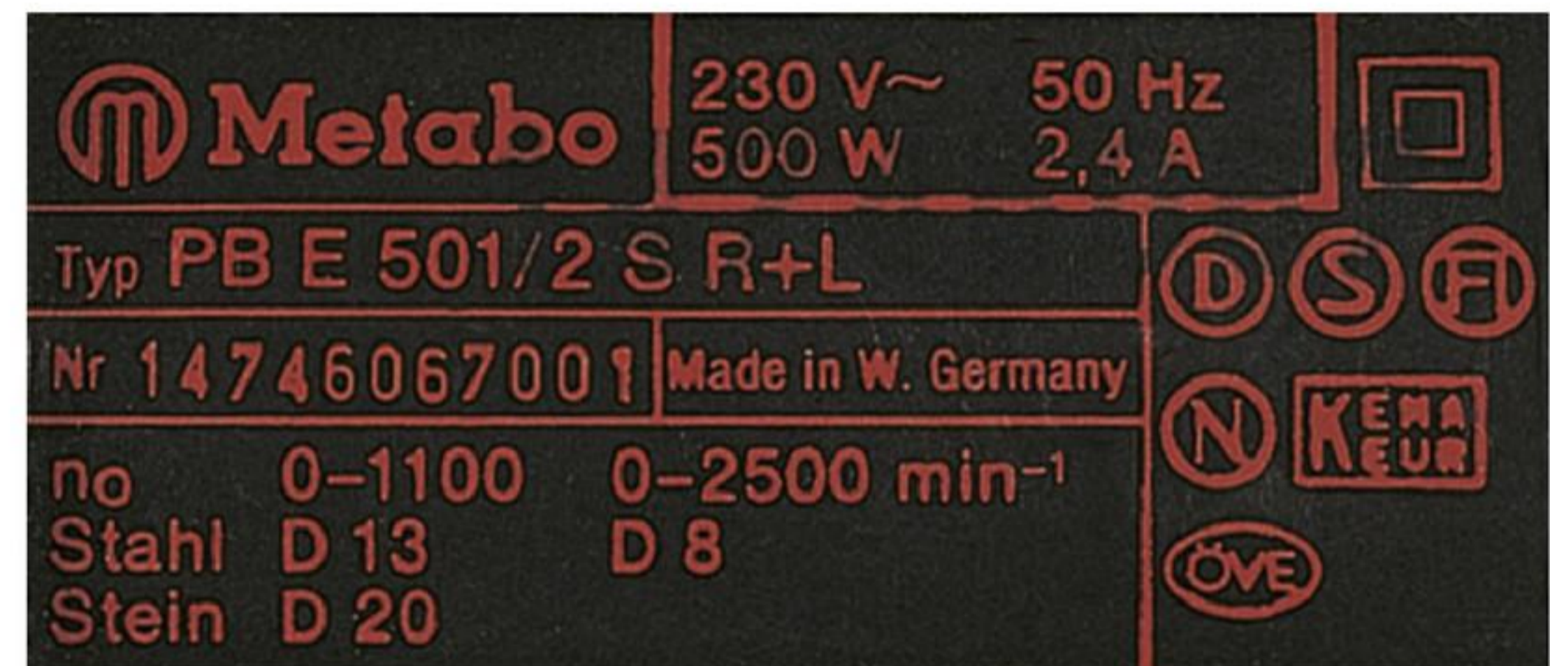
afbeelding 6 Het typeplaatje van een boormachine.
