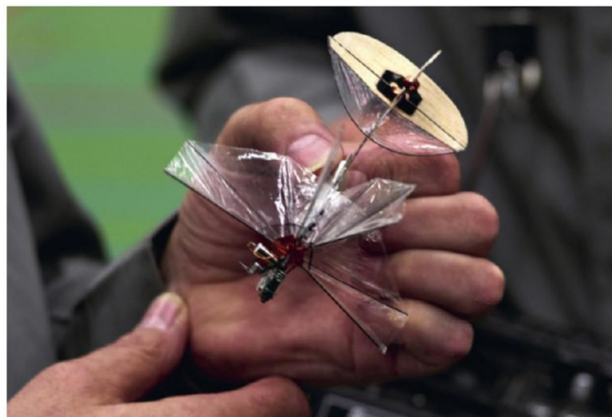
figuur 3 De DelFly Micro .
