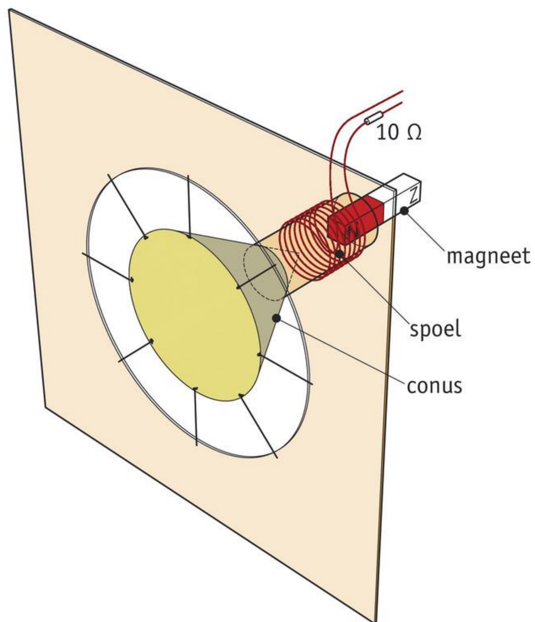
figuur 2 De bouwtekening van een eenvoudige zelfbouwuidspreker.
