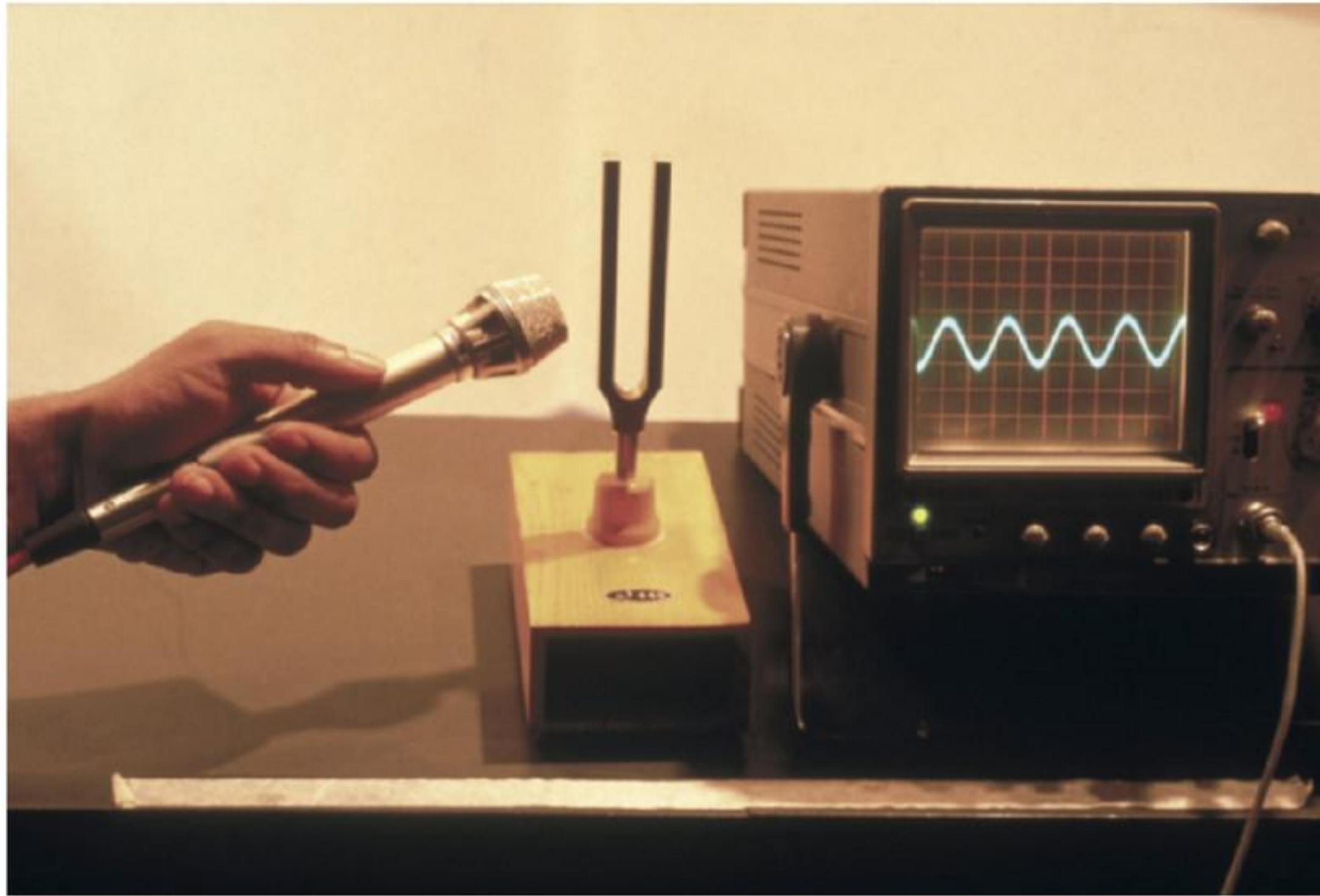
figuur 3 De trilling van een stemvork op een oscilloscoop.
