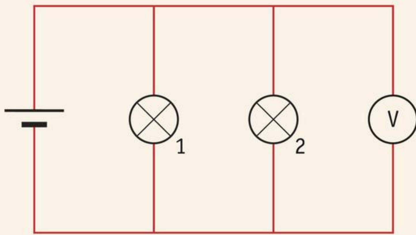
afbeelding 9 Spanning meten over twee parallel geschakelde lampjes.
