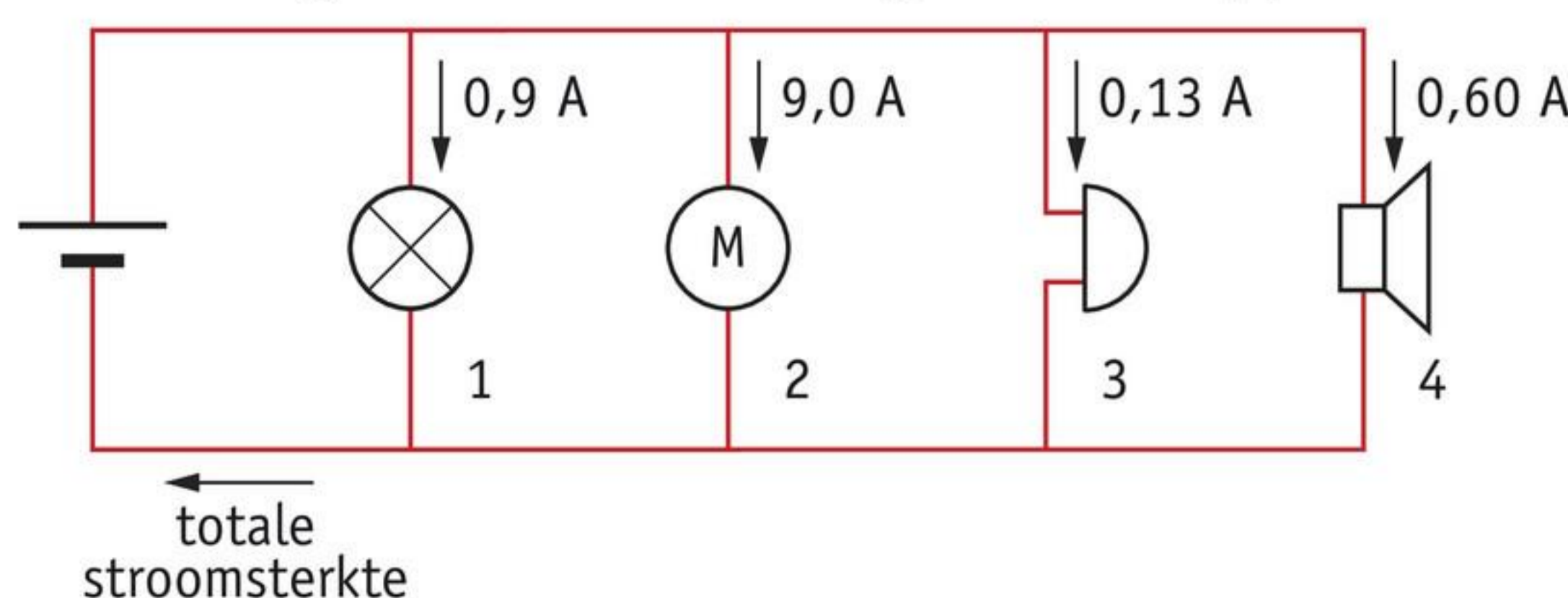
afbeelding 16 Een schakeling met vier apparaten.
