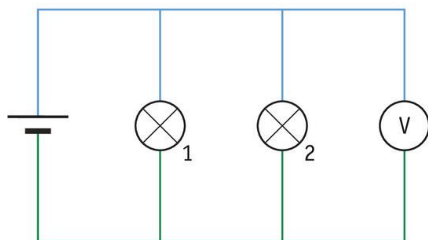
afbeelding 7 Spanning over twee parallel geschakelde lampjes meten.
