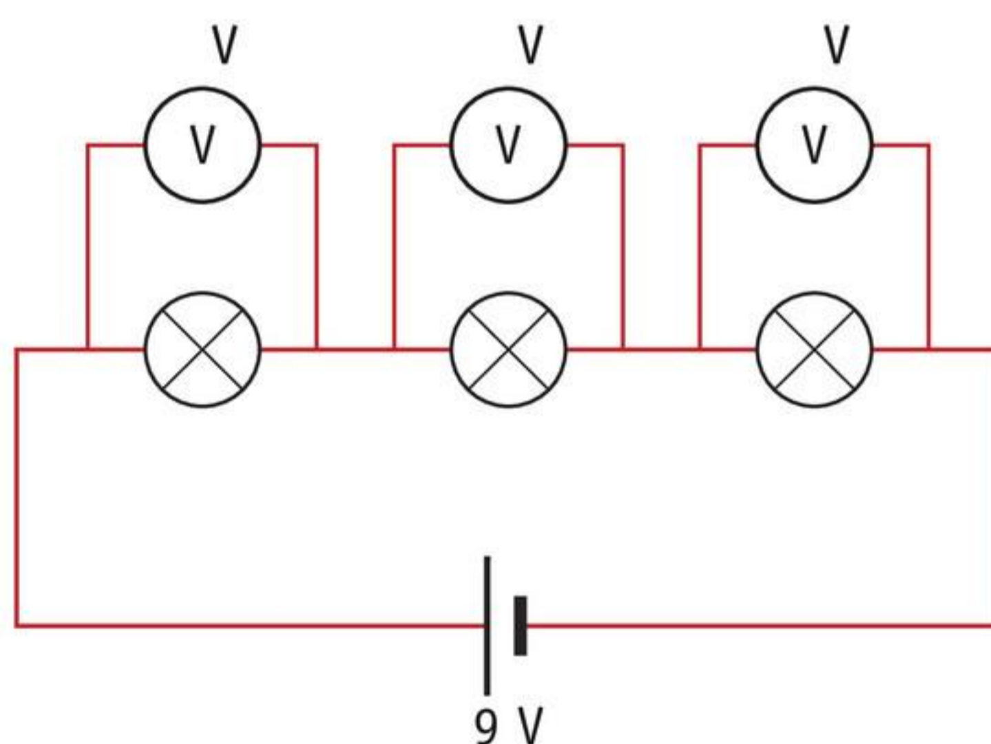
afbeelding 16 Spanning meten over drie lampjes.
