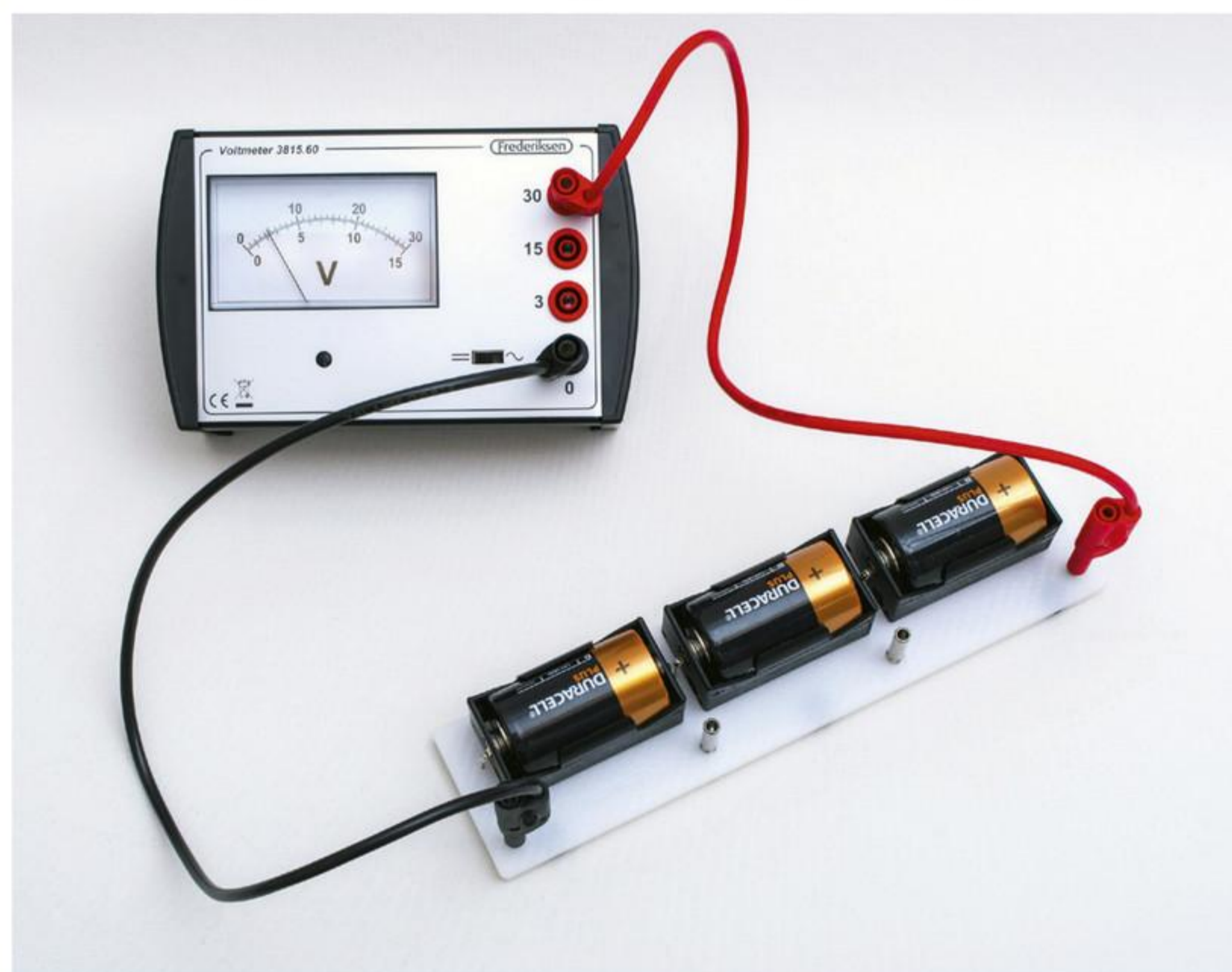
afbeelding 1 Schakeling om de spanning over een batterij te meten.
