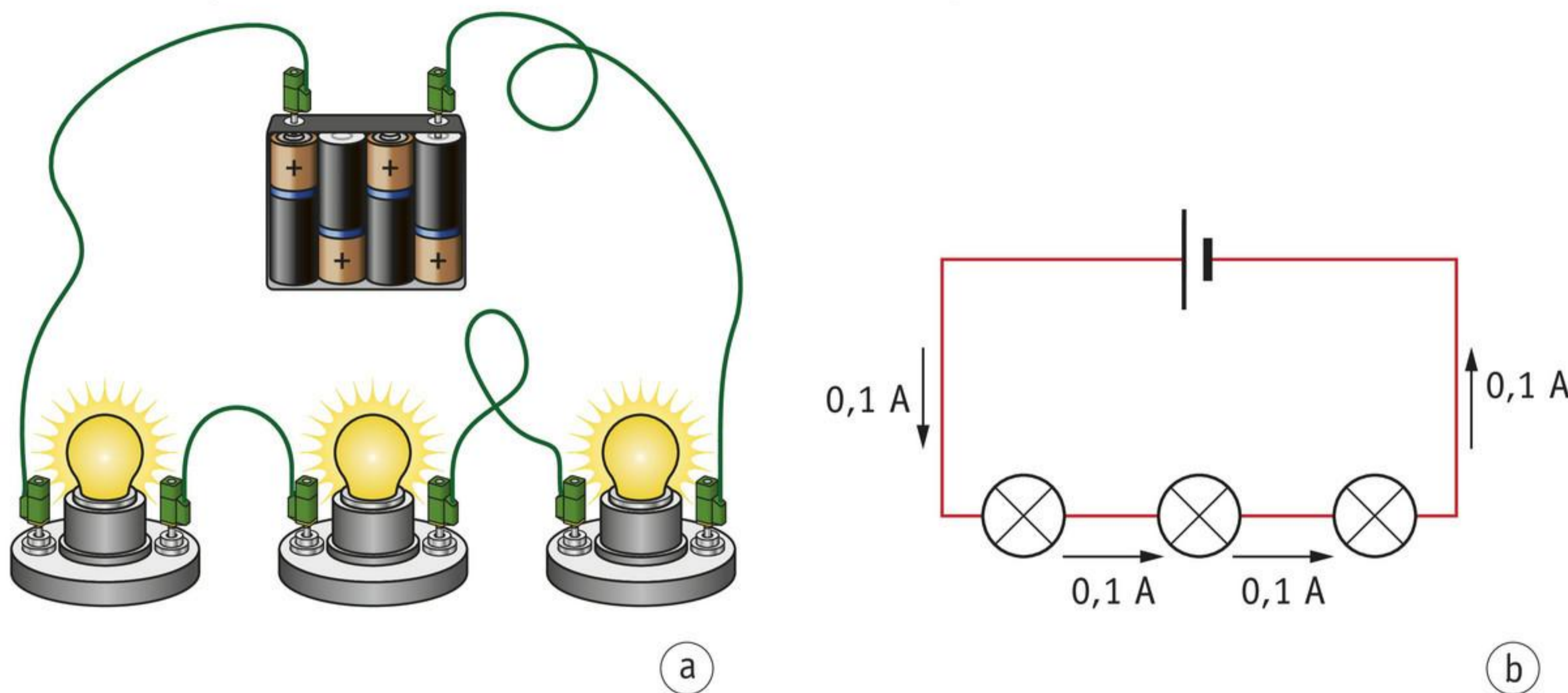
afbeelding 6 De stroomsterkte is overal even groot.
