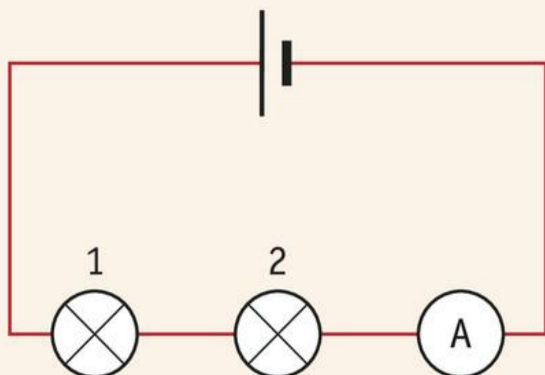
afbeelding 9 Het derde schakelschema van proef 1.
