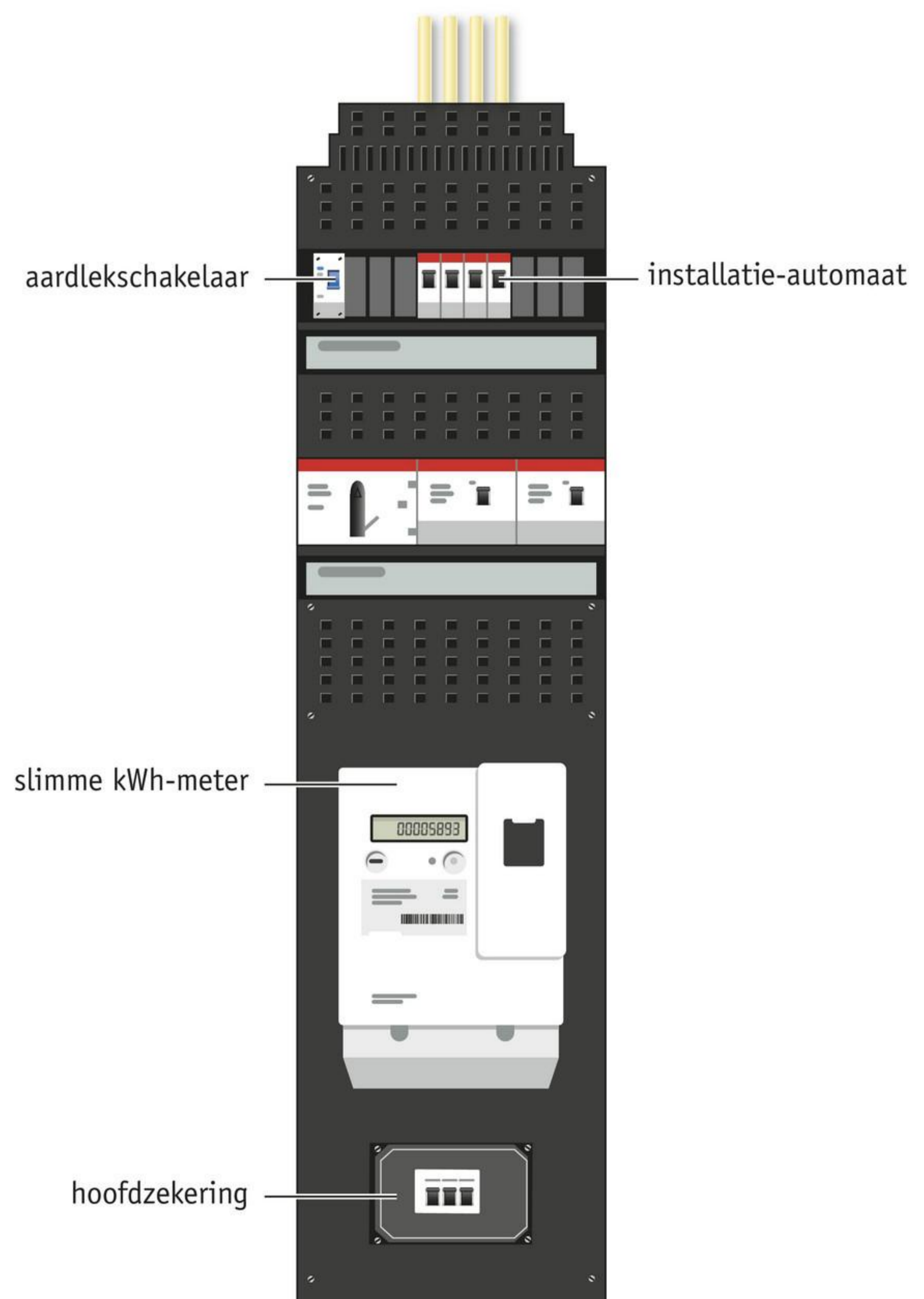
afbeelding 1 De groepenkast in de meterkast.
