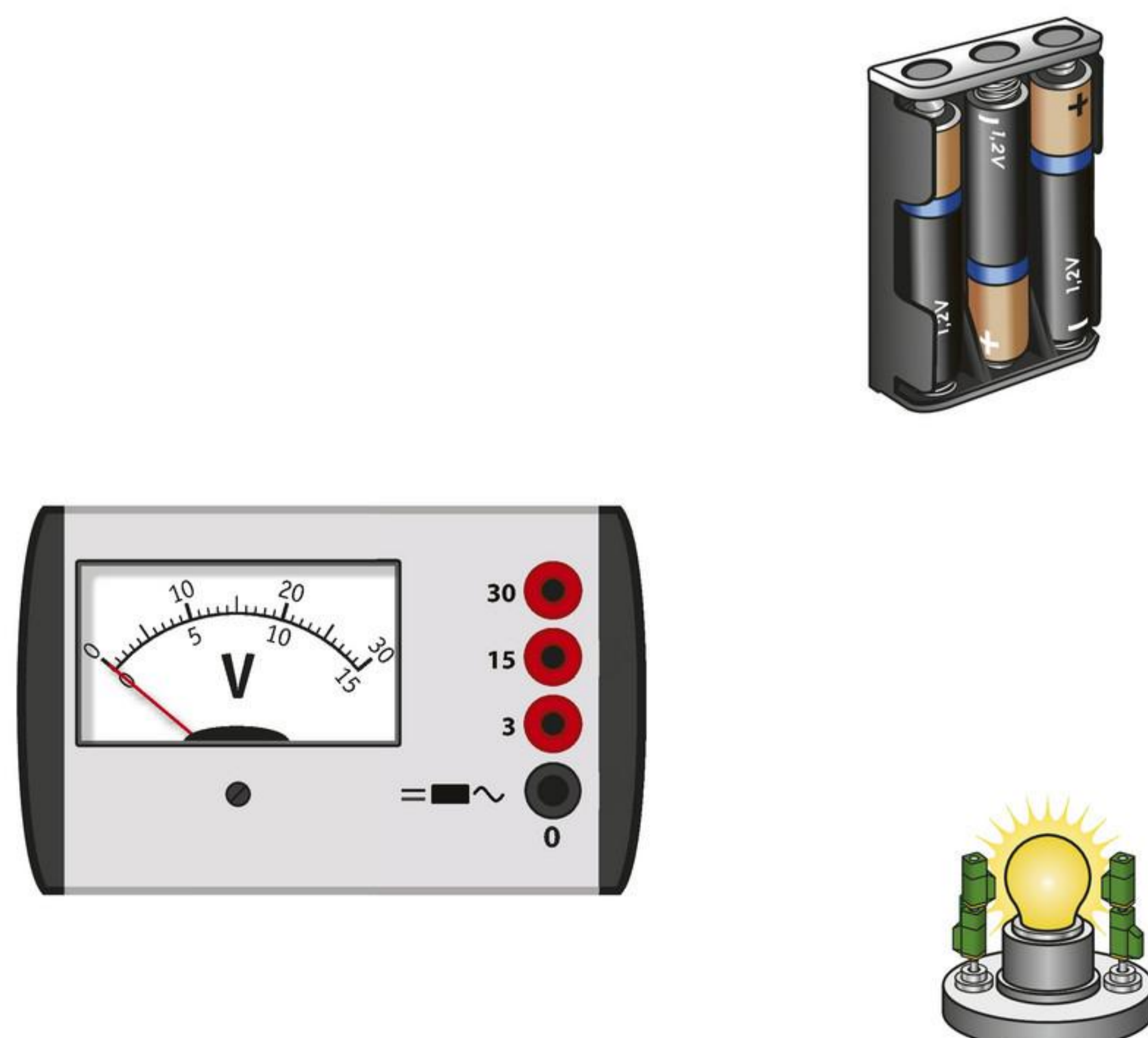
afbeelding 5 Spanning meten over een lampje.
