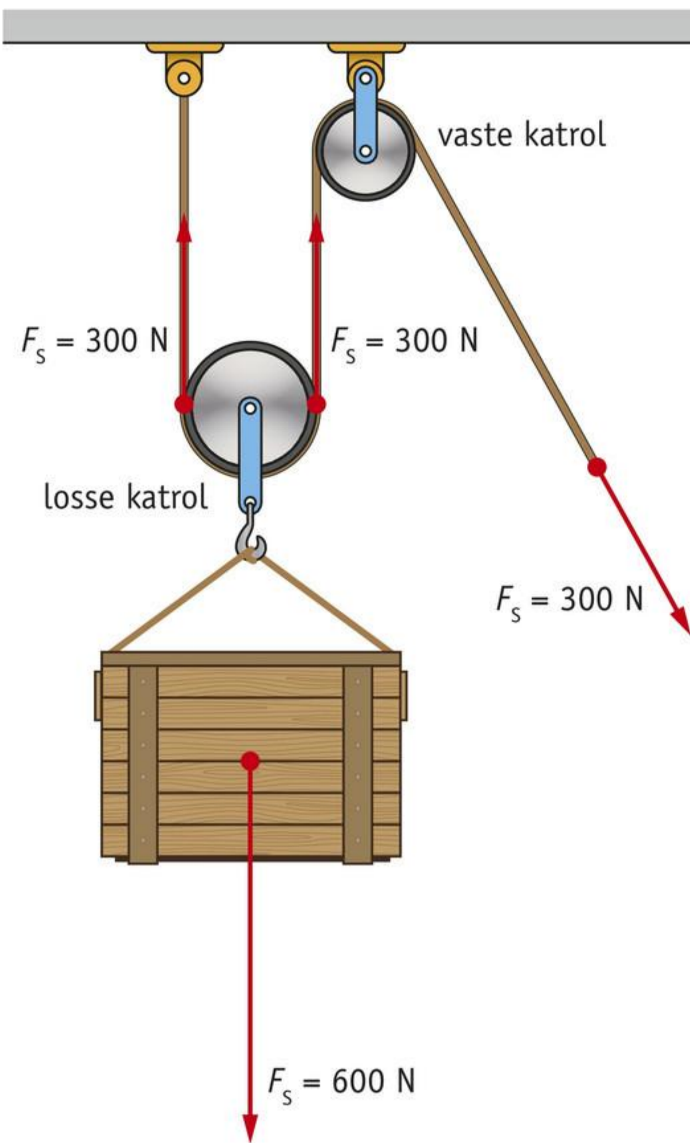
afbeelding 9 De kracht is verdeeld over twee stukken touw.
