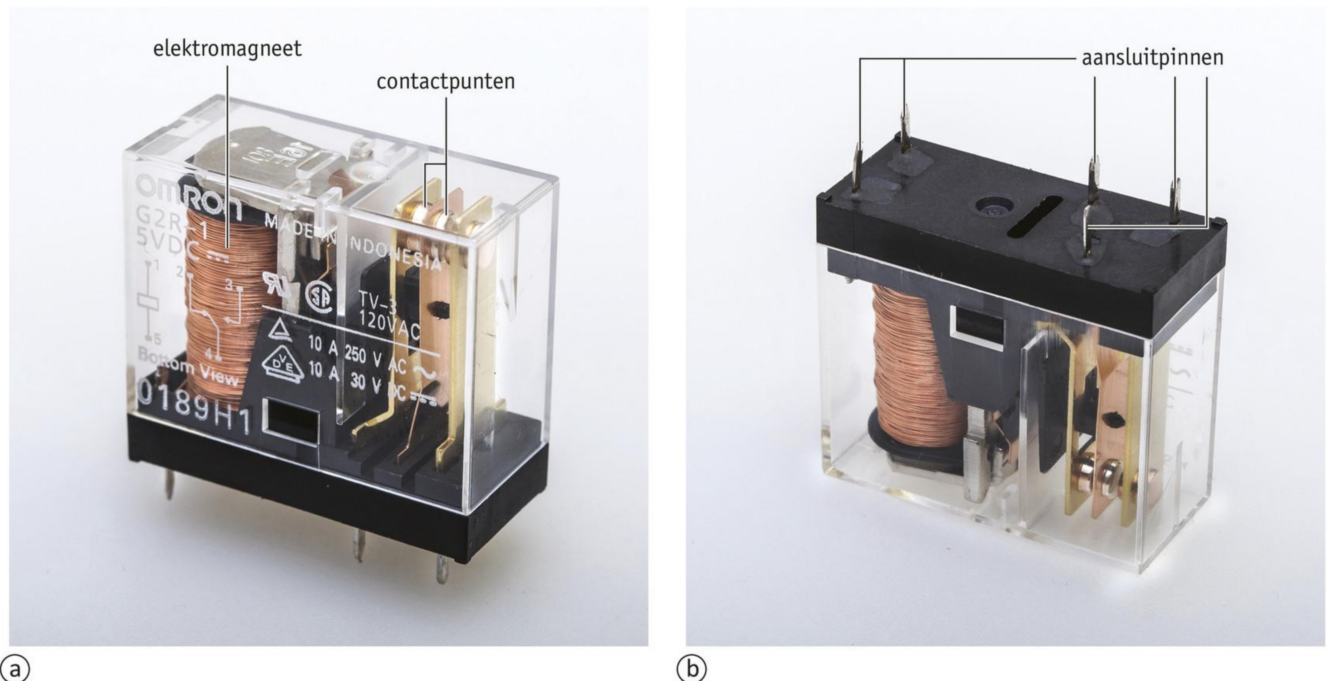
afbeelding 3 Een relais: van boven (a) en van onderen (b).
