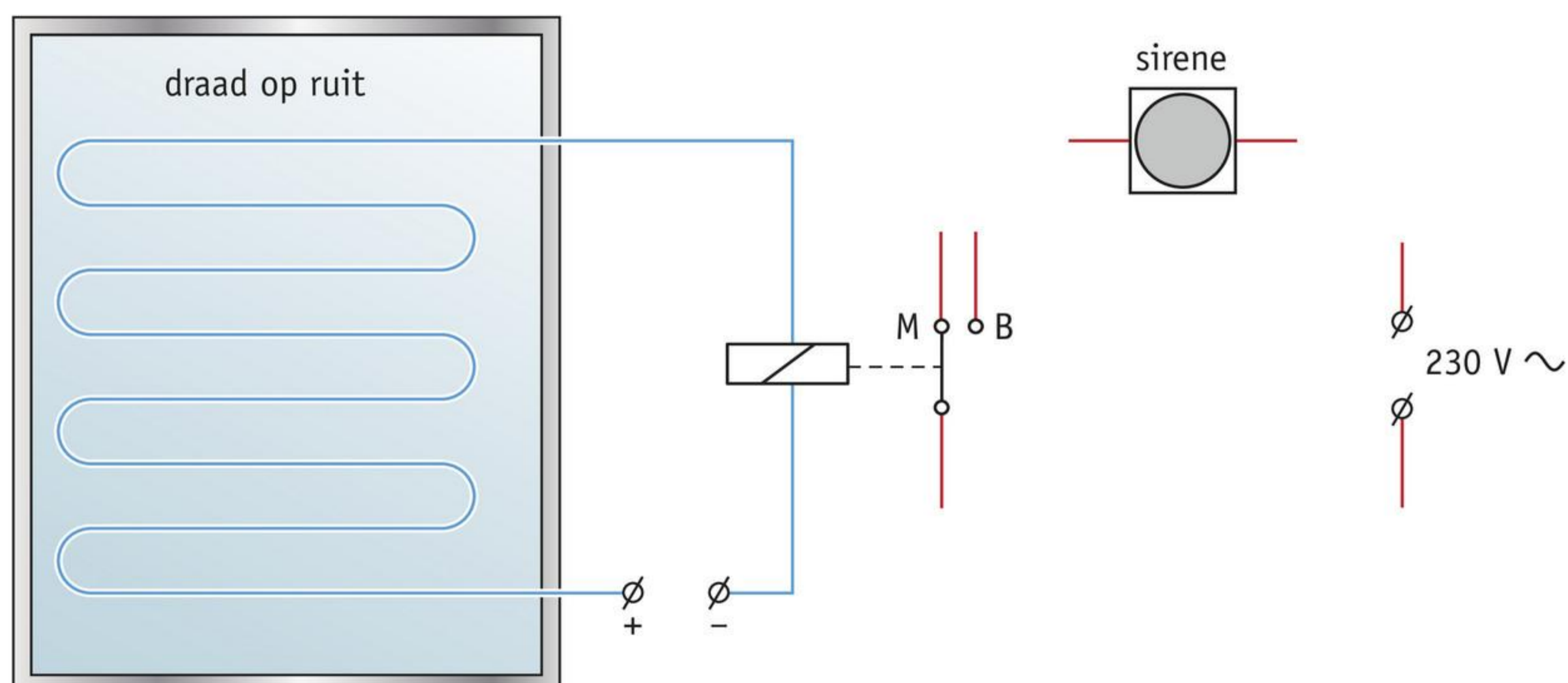
afbeelding 8 Een inbraakalarm.
