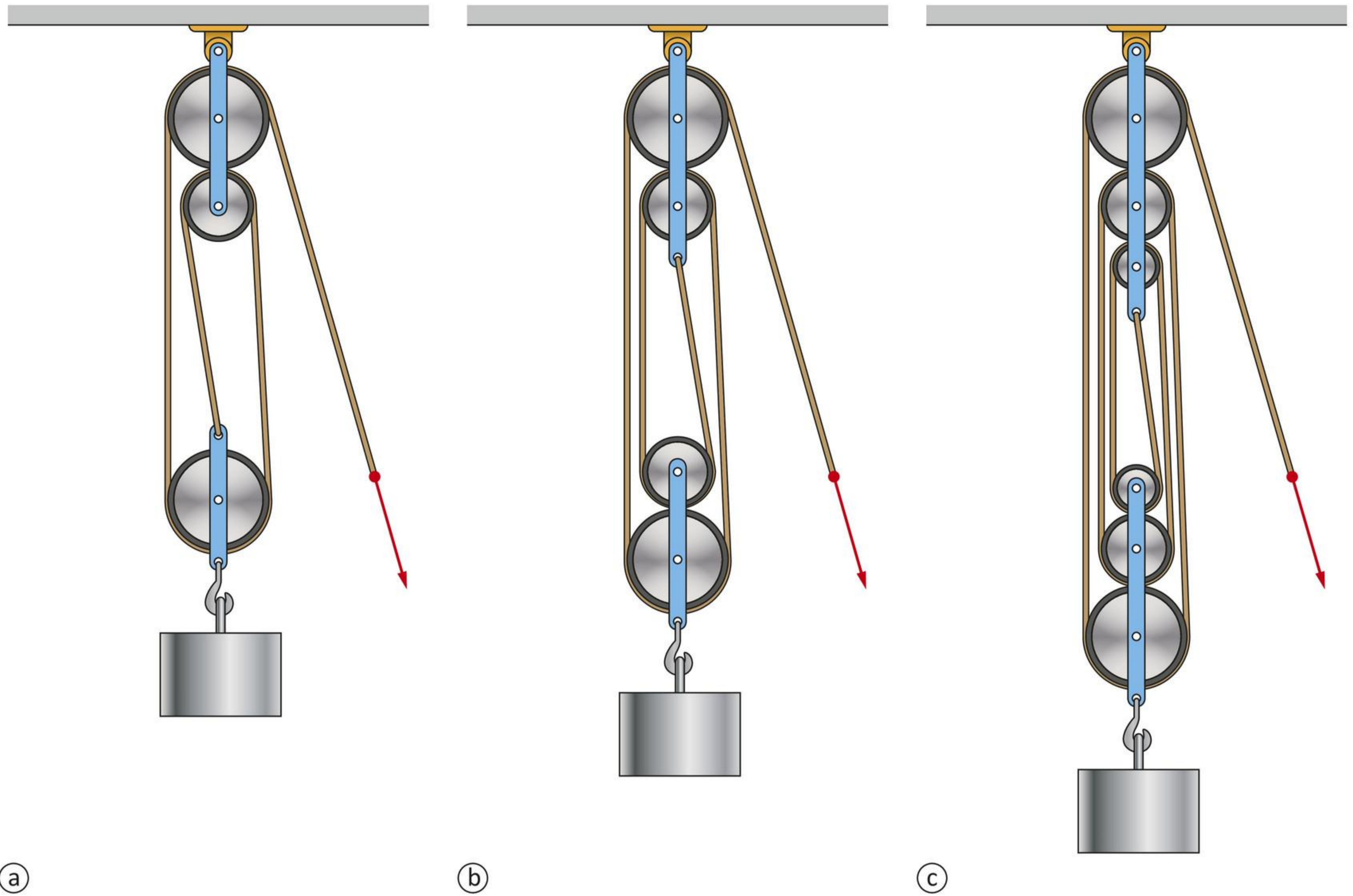
afbeelding 13 Drie takels.
