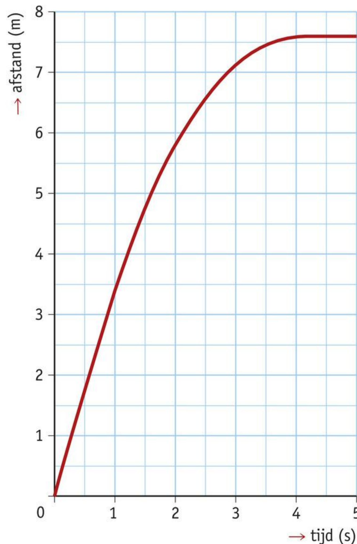
b een vertraagde beweging
