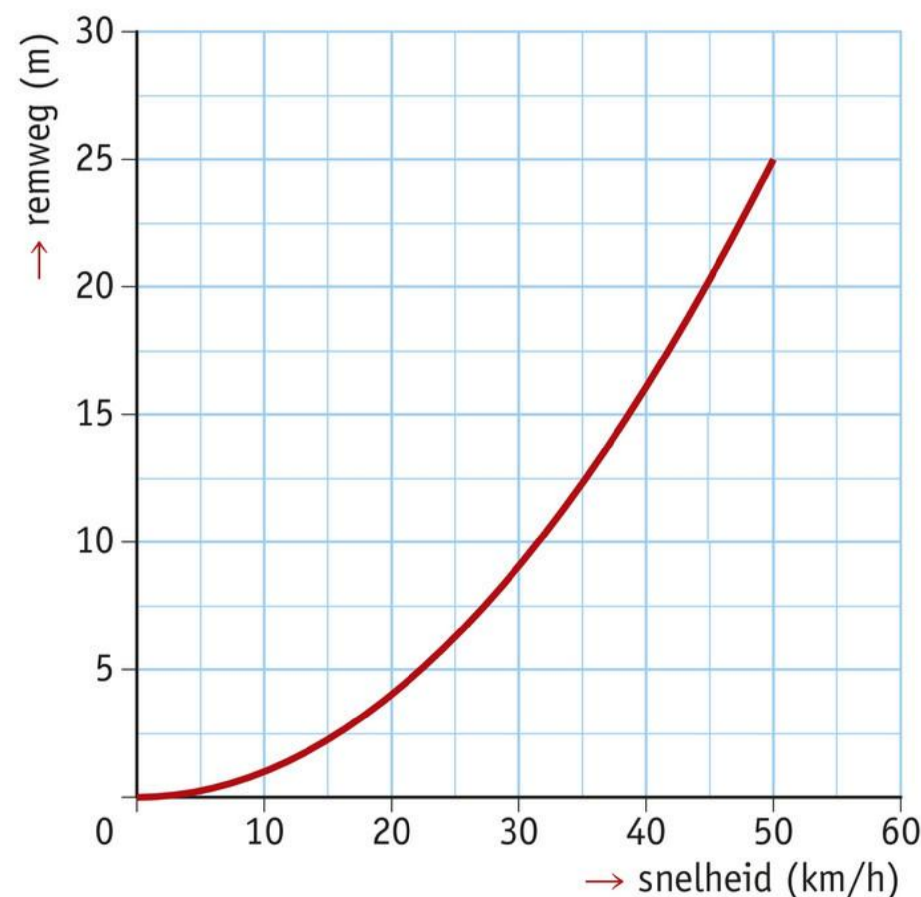
afbeelding 4 De grafiek van de remweg van een scooter.
