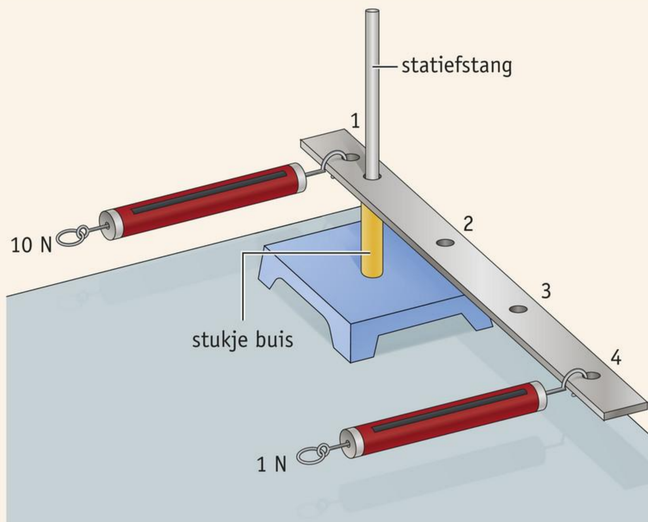
afbeelding 6 De opstelling van proef 1.
