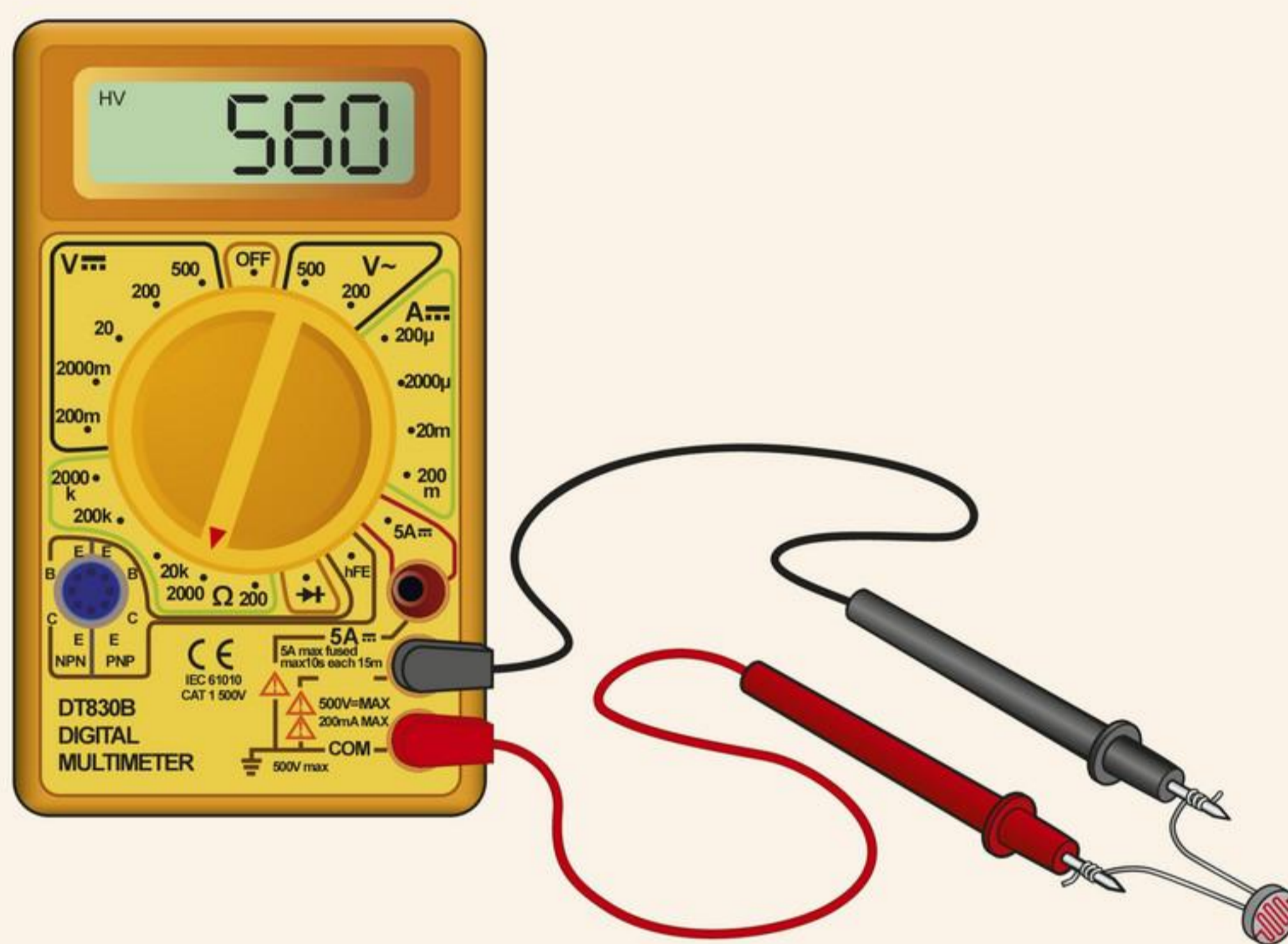
afbeelding 8 Aansluiting van een LDR op een multimeter.
