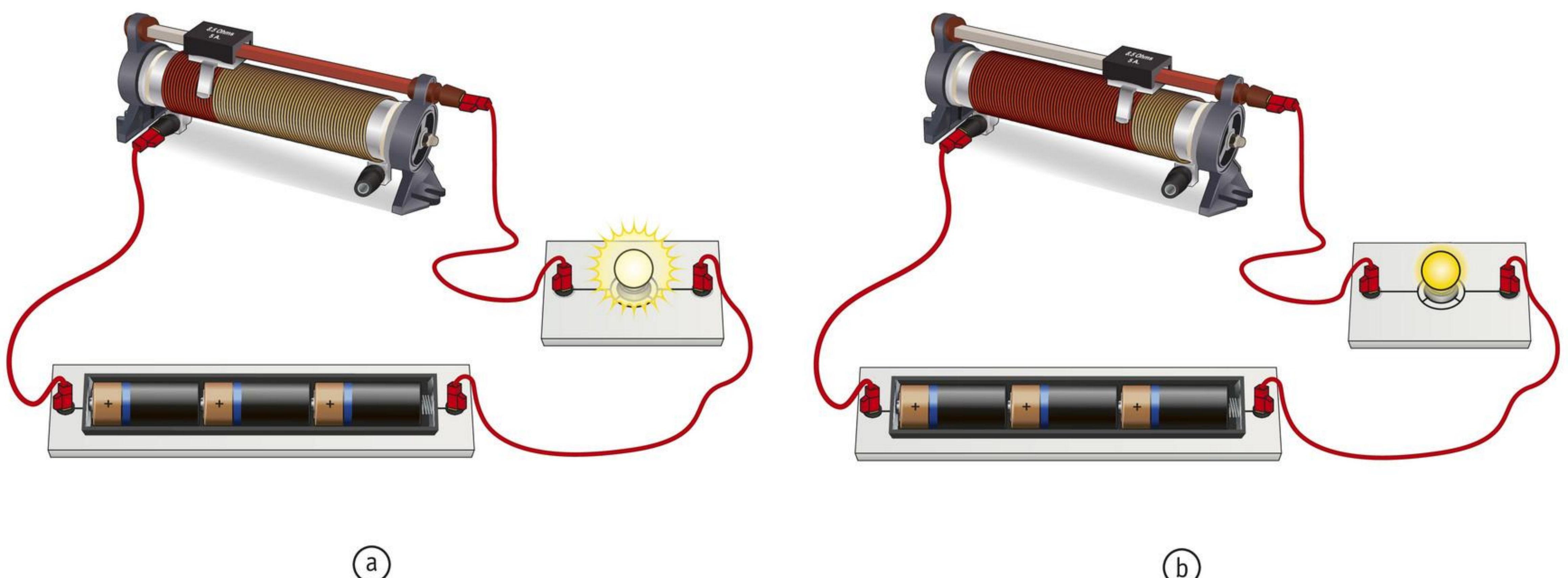
afbeelding 12 Zo werkt een schuifweerstand.
