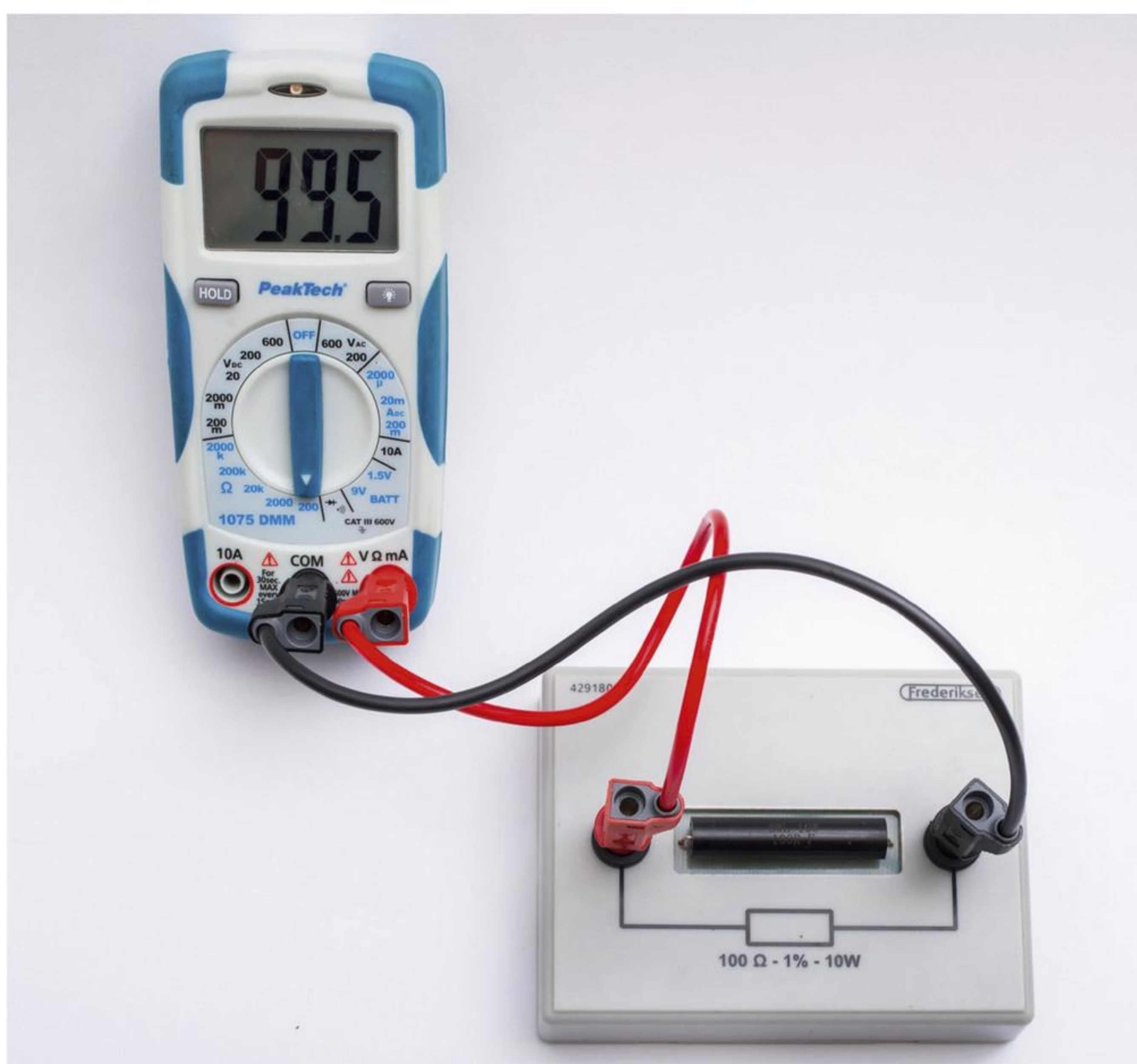
afbeelding 6 Weerstand meten met een multimeter.
