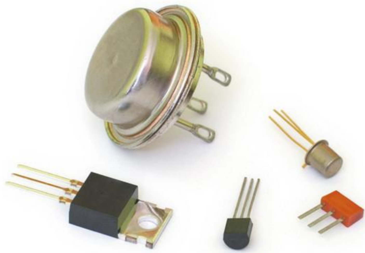
afbeelding 13 Verschillende transistors.
