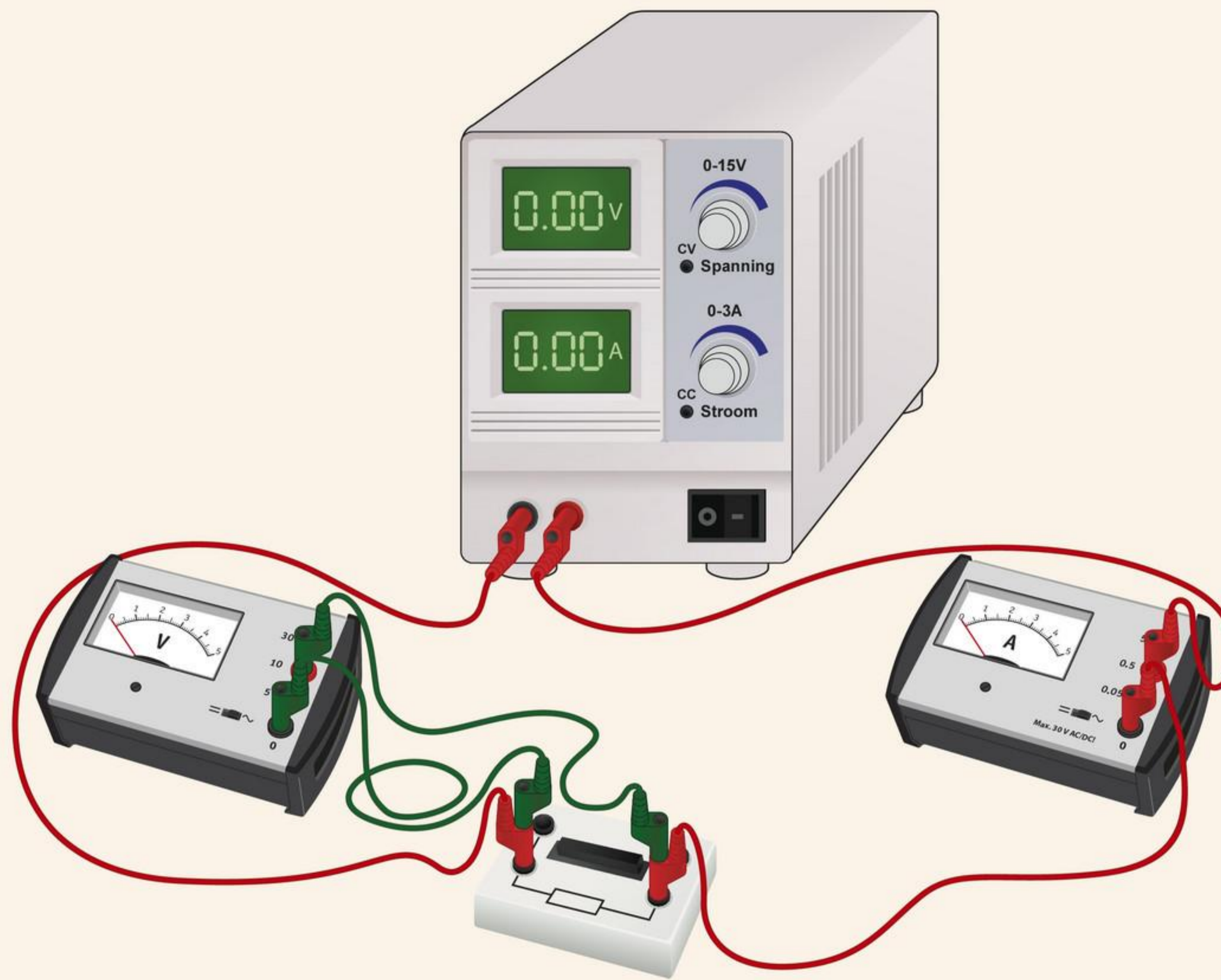
afbeelding 5 De aansluiting voor de meting.
