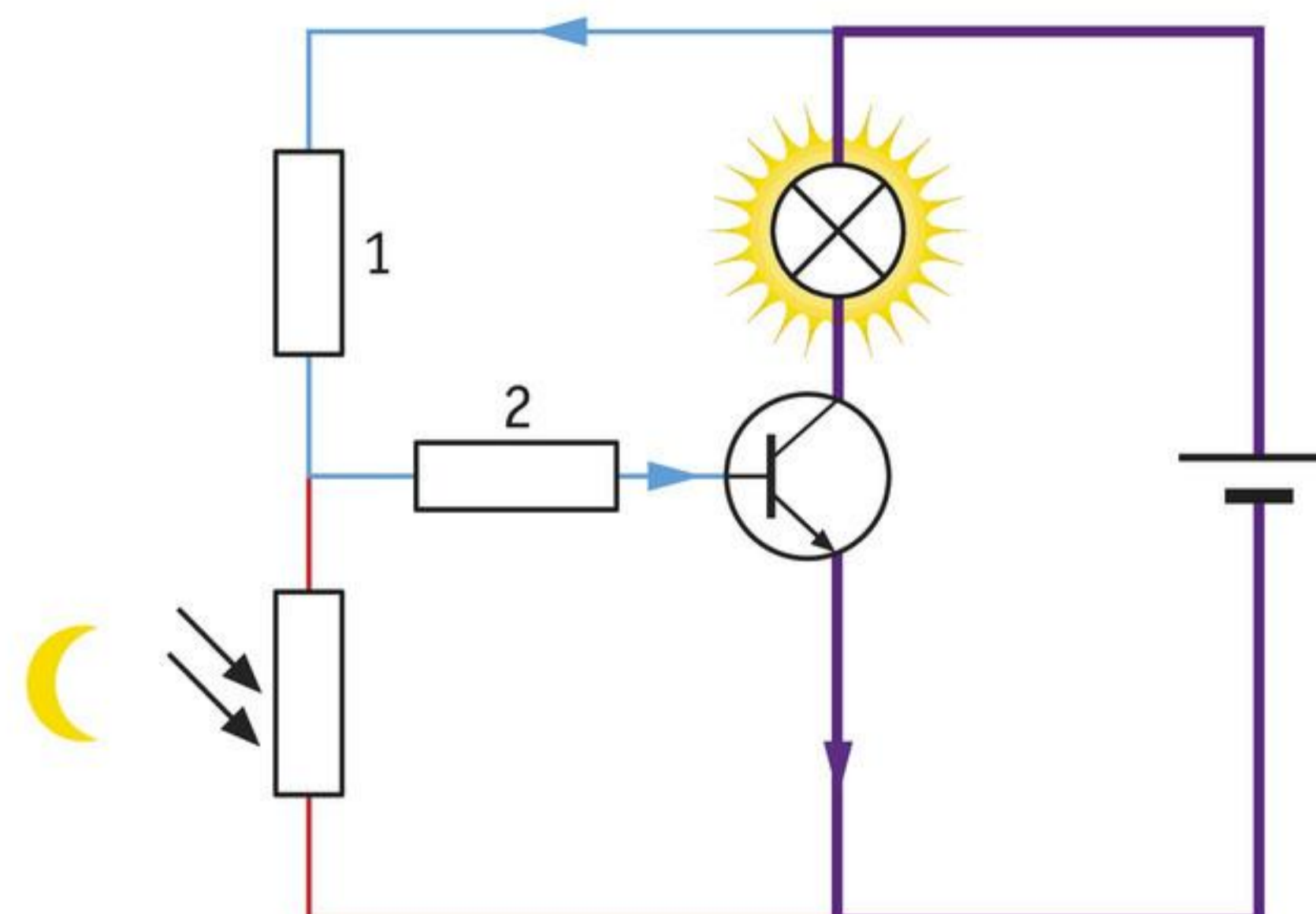
b Er loopt nu een klein stroompje via de basis; de transistor staat in de AAN-stand.
