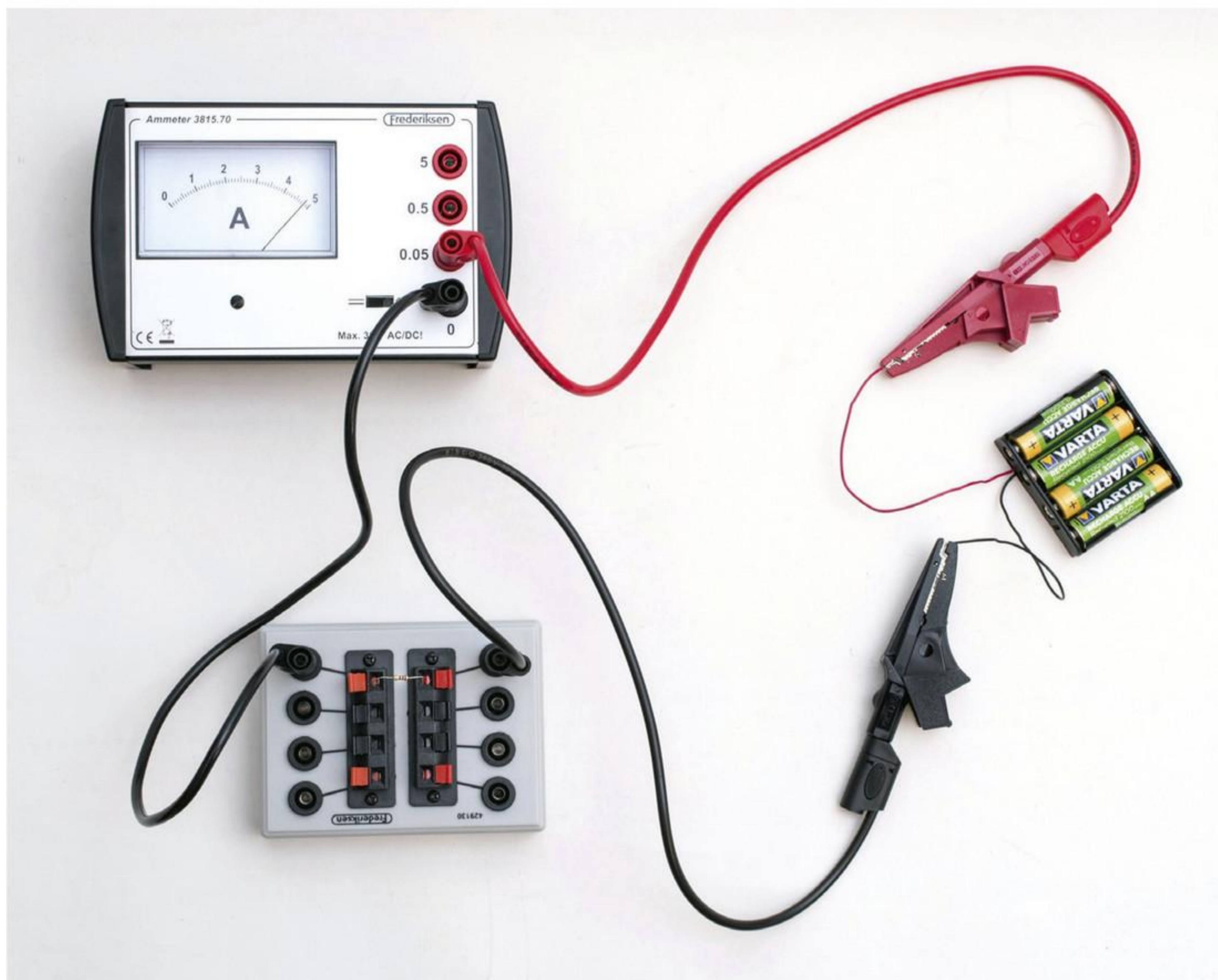
afbeelding 4 Schakeling met stroommeter en weerstand.
