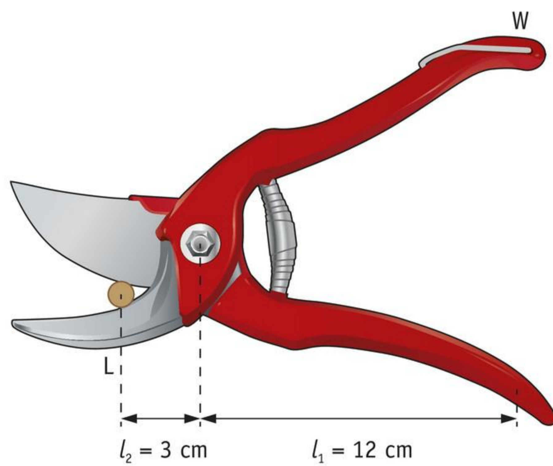
afbeelding 10 Met een snoeischaar knijpt Janice een takje door.
