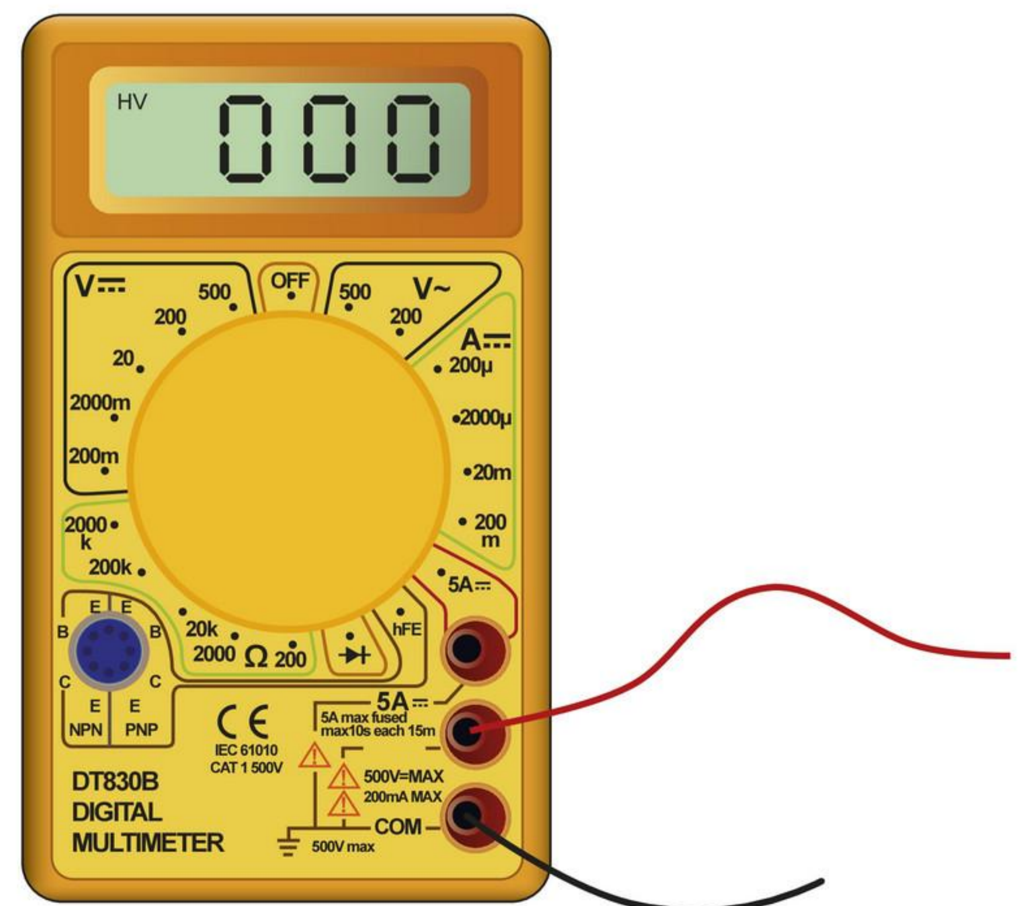
afbeelding 10 De multimeter gebruiken als stroommeter.
