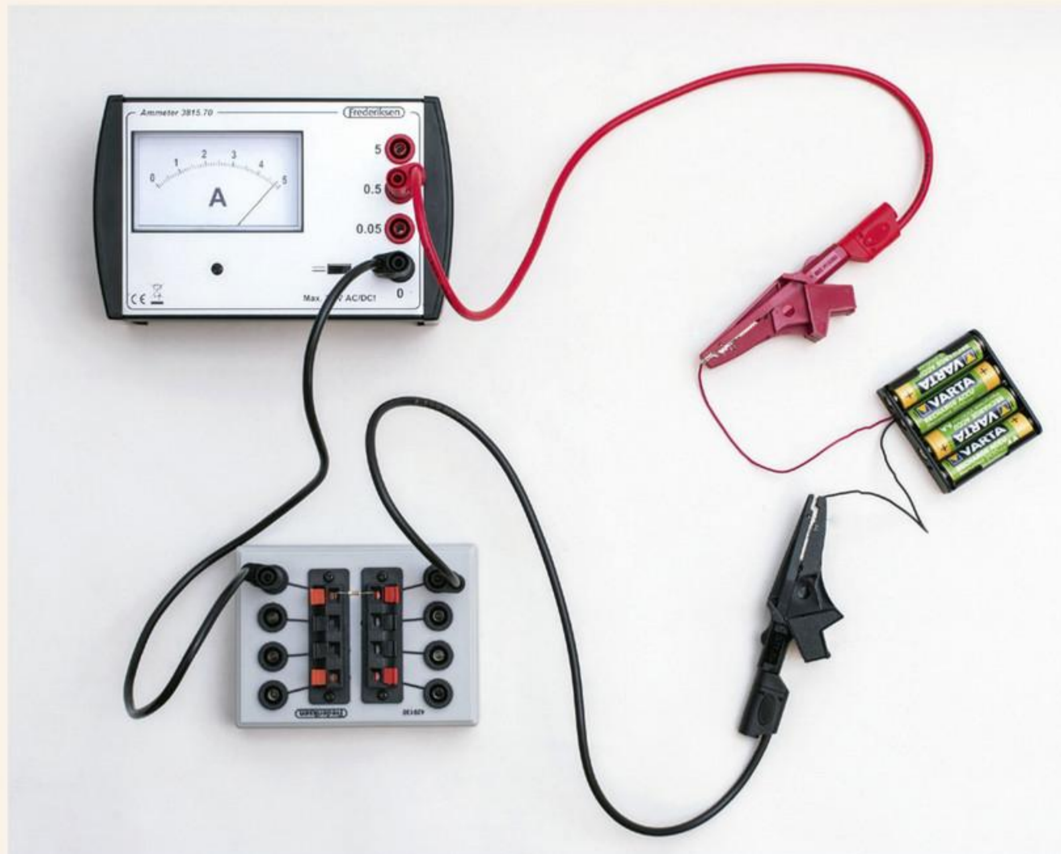
afbeelding 3 Meten van de stroomsterkte door één weerstand.
