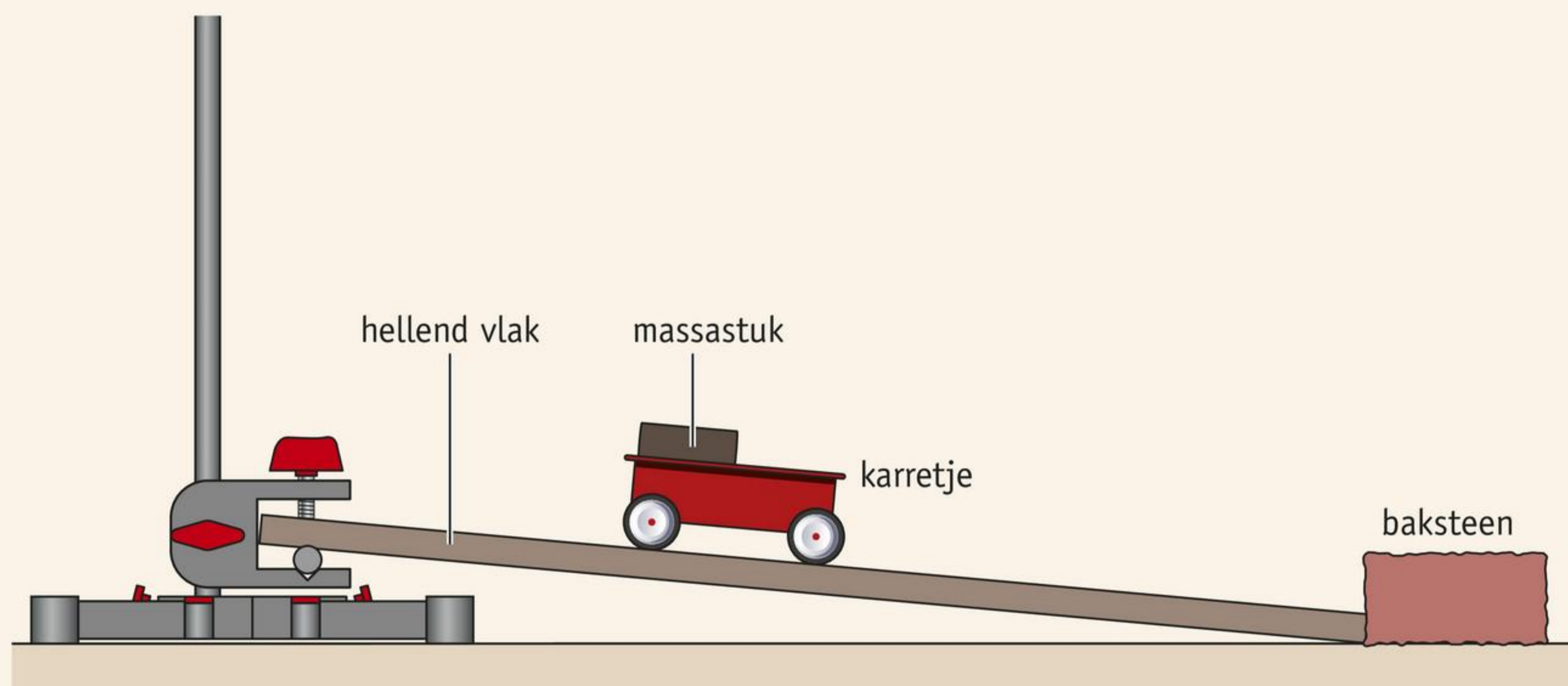
afbeelding 5 De opstelling van proef 1.
