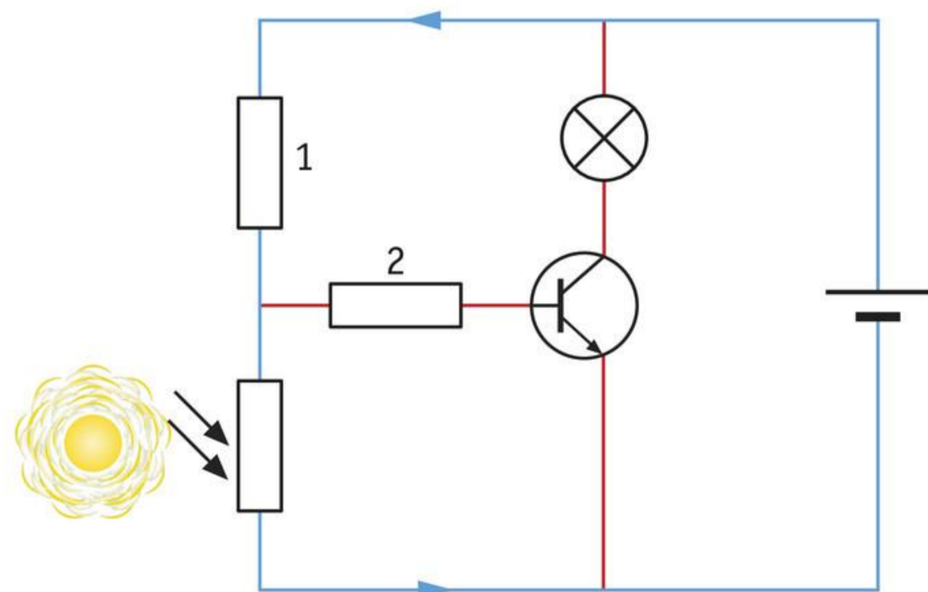
a Bijna alle stroom loopt via de LDR; de transistor staat in de UIT-stand.
